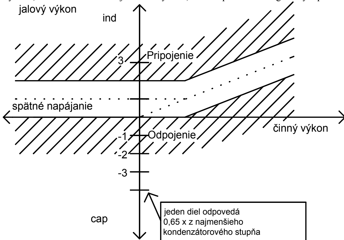
Obr. 8: Regulačné pásmo pri nastavení cieľového \cos \varphi = 0,92 ind; L = +1,0
