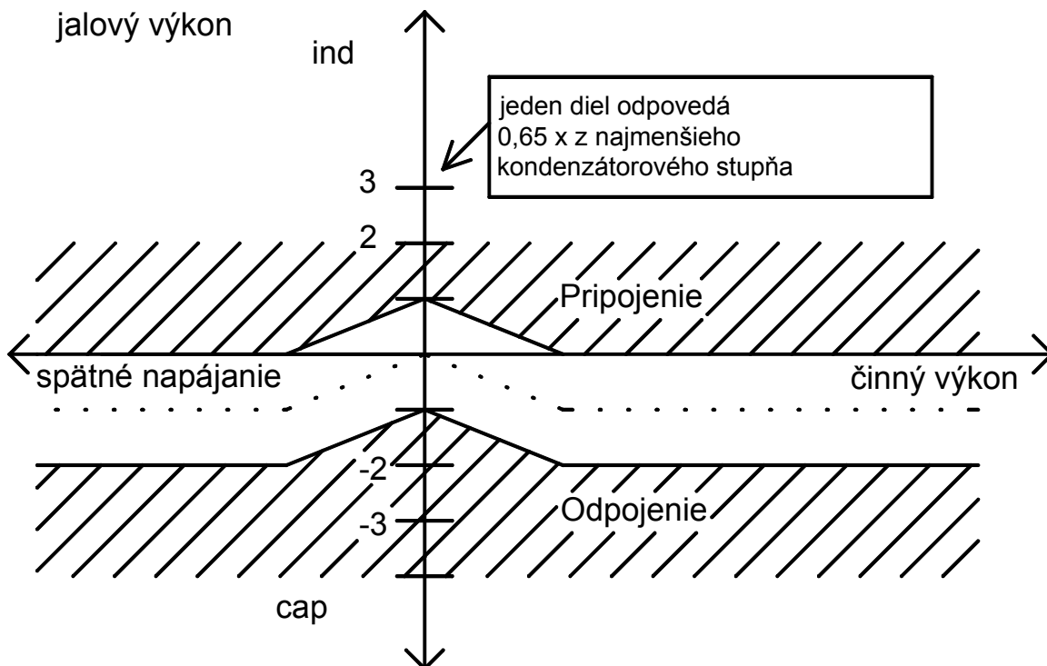
Obr. 10: Regulačné pásmo pri nastavení cieľového \cos \varphi = 0,95 cap; PS = 0; L = -1,0
