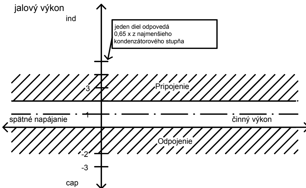
Obr. 6: Regulačné pásmo pri nastavení cieľového \cos \varphi = 1 ; PS = +1,0 ; L = OFF
