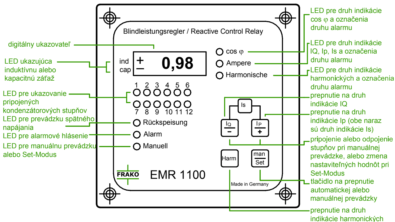
Obr. 1: Pohľad spredu
