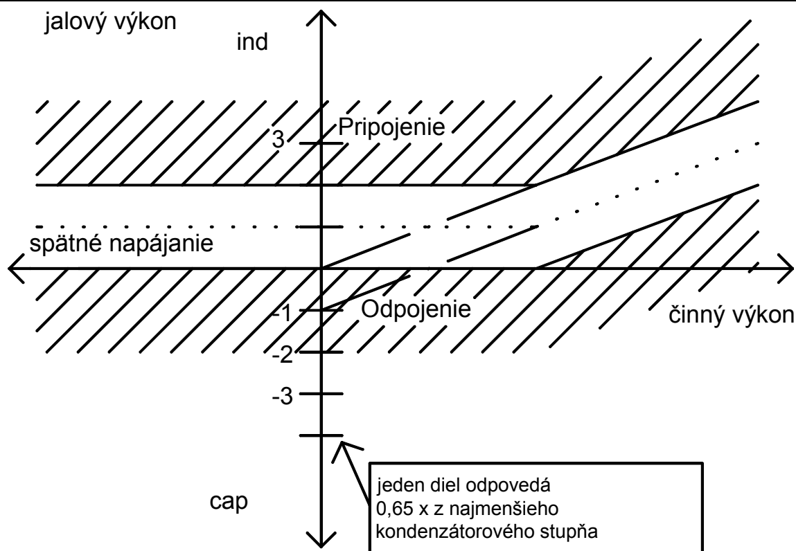
Obr. 9: Regulačné pásmo pri nastavení cieľového \cos \varphi = 0,92 ind; PS = -1,0; L = +1,0
