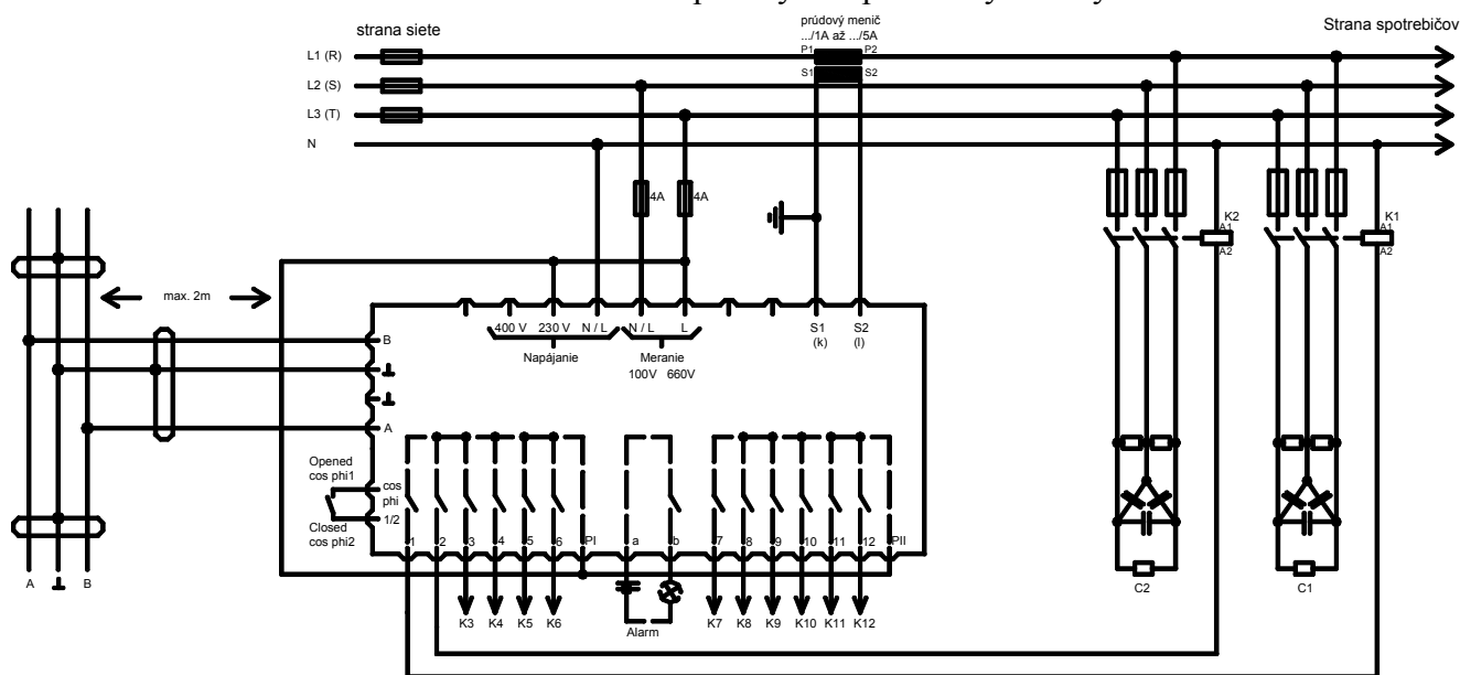
Obr. 3: Pripojenie
