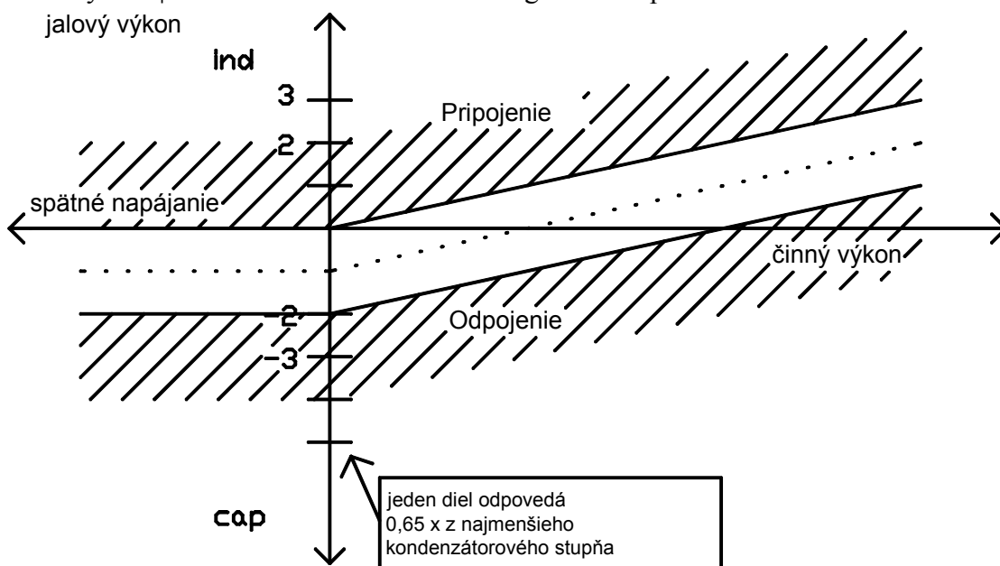
Obr. 7: Regulačné pásmo pri nastavení cieľového \cos \varphi = 0,92 ind; PS = -1,0 ; L = OFF
