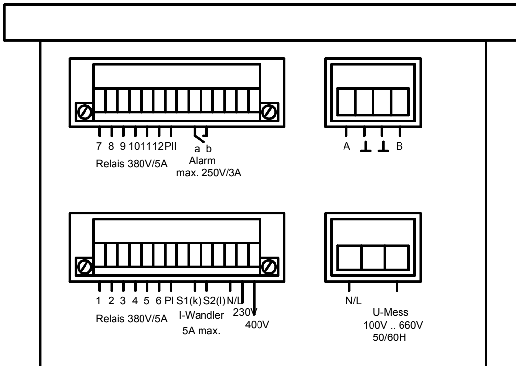
Obr. 2: Pohľad zospodu
