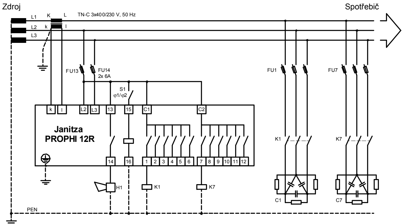
Příklad zapojení regulátoru účinníku s 12 reléovými výstupy, přepínačem cílové hodnoty \cos \varphi a alarmovým výstupem
